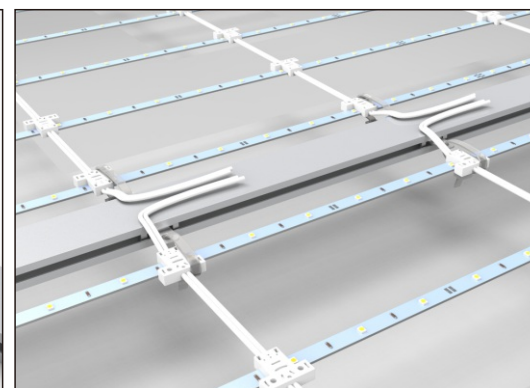
双面灯箱框架组装完成图
