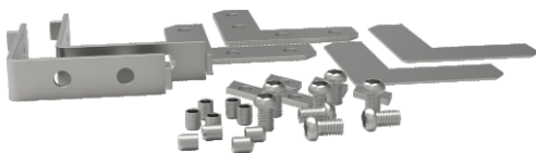
小角码N-4个 大角码M-4个+垫片
