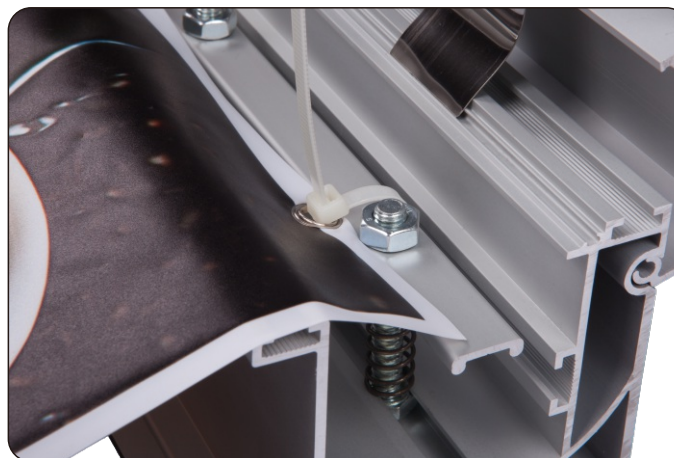
画面固定方式——弹簧铝条挤压式
