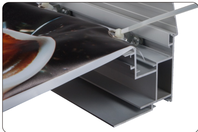
画面固定方式——简易滑扣式
