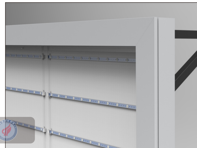
3.将漫反射LED灯固定至背板
