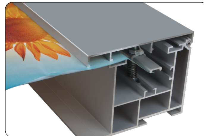
画面固定方式——弹簧铝条挤压式
