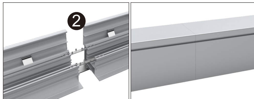
2.按②图示对超过6米的铝材进行接驳拼接。
