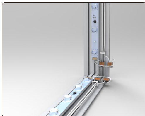
② 在铝材内安装侧光源（自选）
