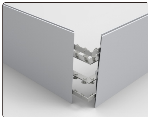
① 四个直角拼接方式
