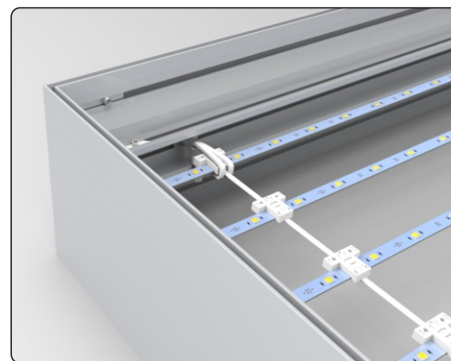
③ 在铝材内安装双面背光源(自选)
